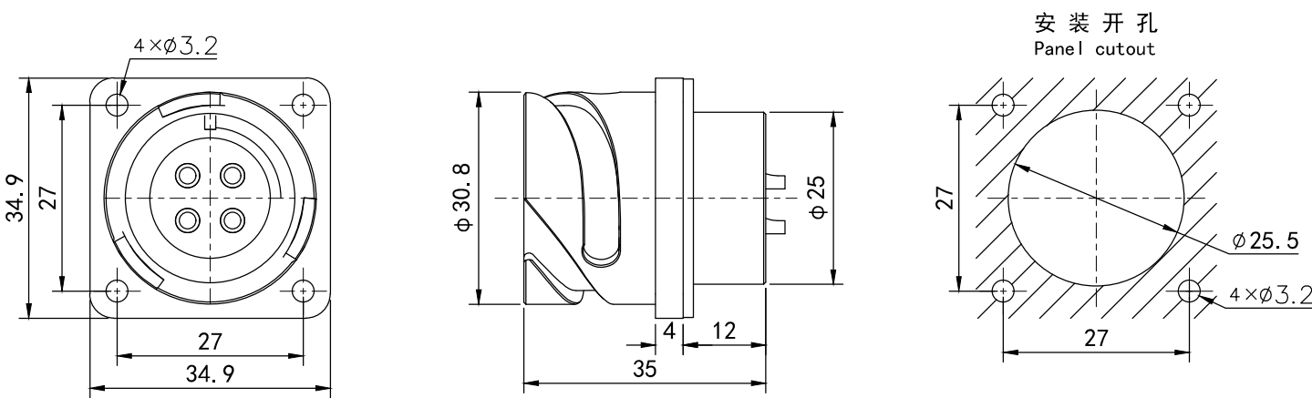
方形法兰插座 Square flange mount receptacle
