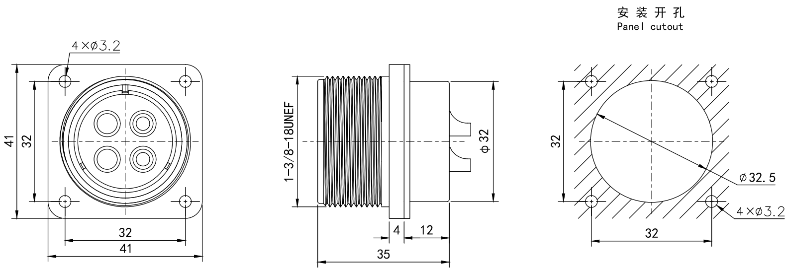
方形法兰插座 Square flange mount receptacle
