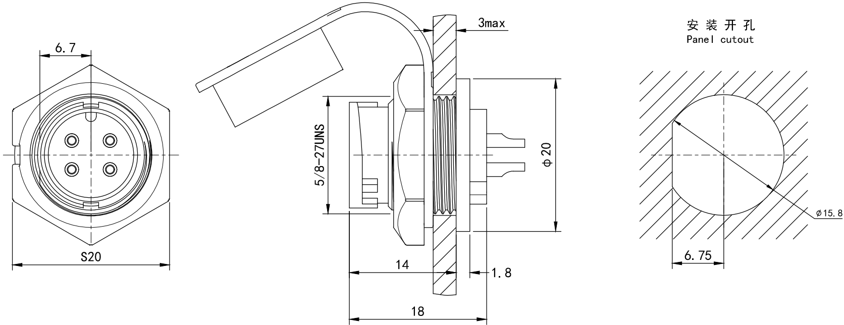
前螺母单切面卡扣插座 Front nut single cut buckle receptacle
