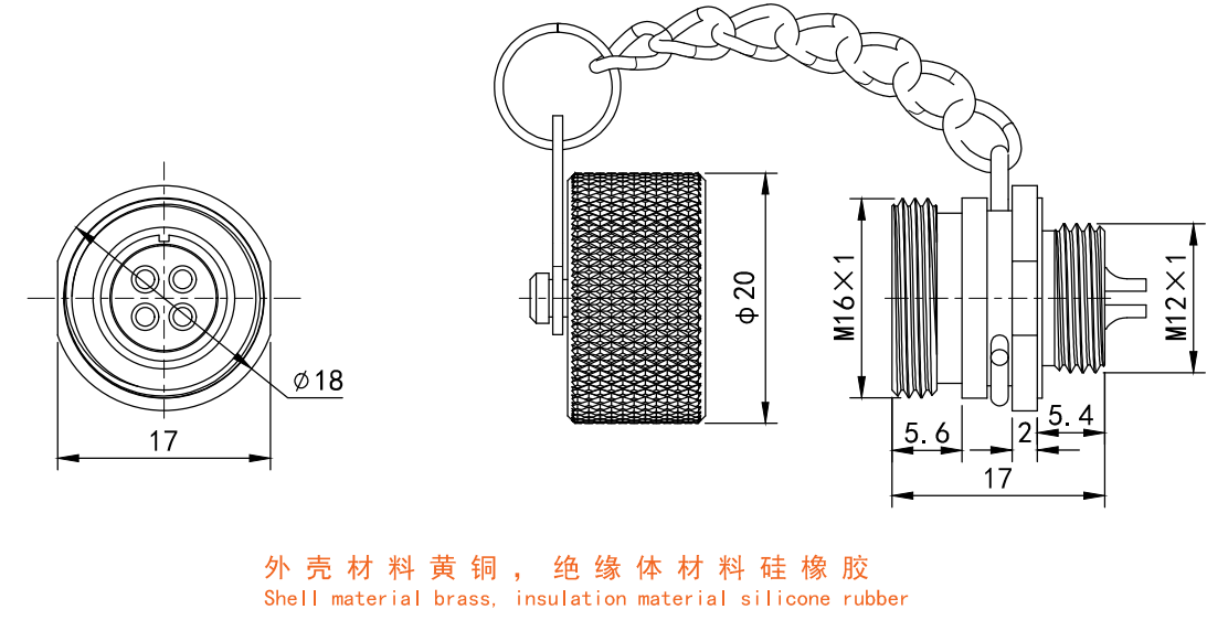
HKCT-80圆形插座 HKCT-80 round receptacle
