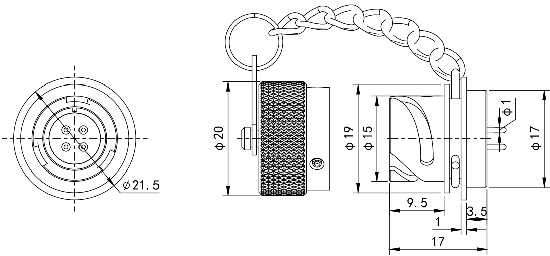
D型卡扣圆形插座 D-type buckle round receptacle
