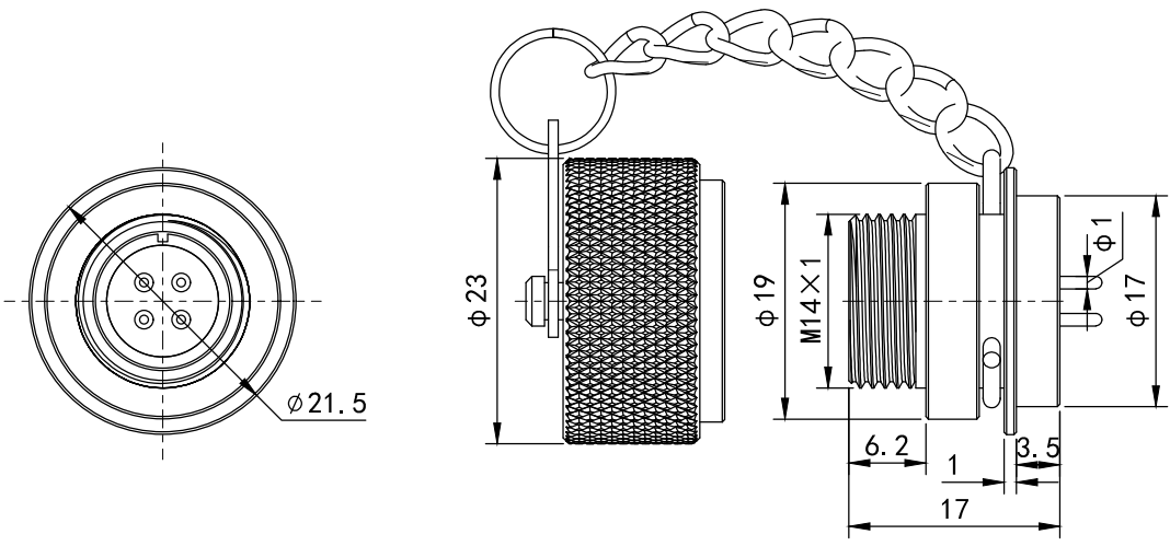
圆形插座 Round receptacle
