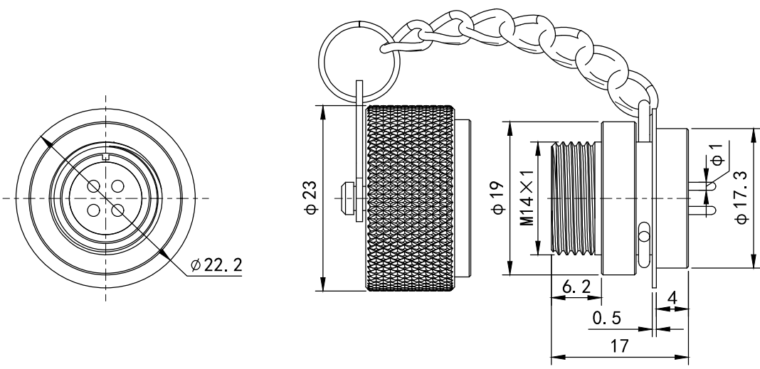
C型圆形插座 C-type round receptacle
